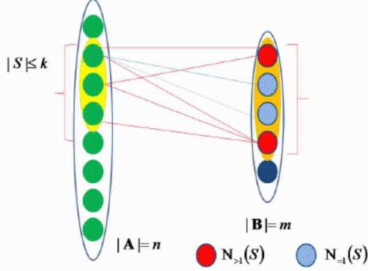
Fig. 2. Progress Lemma
